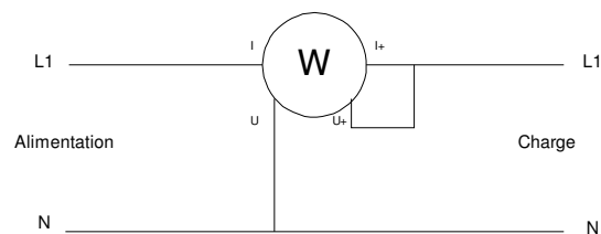
Fig 4.4.1 Schéma de branchement en monophasé
